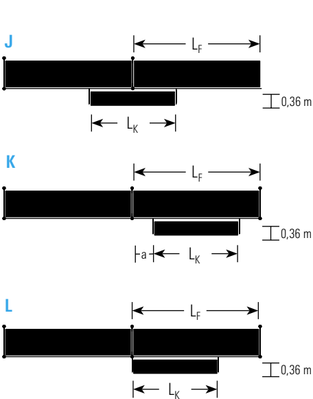
Användning av "böjd" nischkonsol, 0,36 m (Art nr 4006.036)
